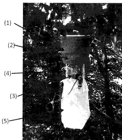
Figura 1: trappola tipo CDC modificata a CO 2 .
